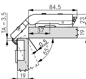
Толщина двери (TS) 19 мм (заводская регулировка) Расстояние до чашки (ТА) 3.5 мм Высота ответной планки 0
